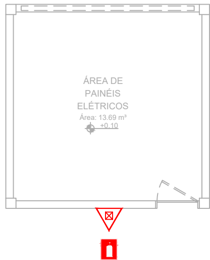
Planta Baixa – Área de Painéis Elétricos escala 1/75
