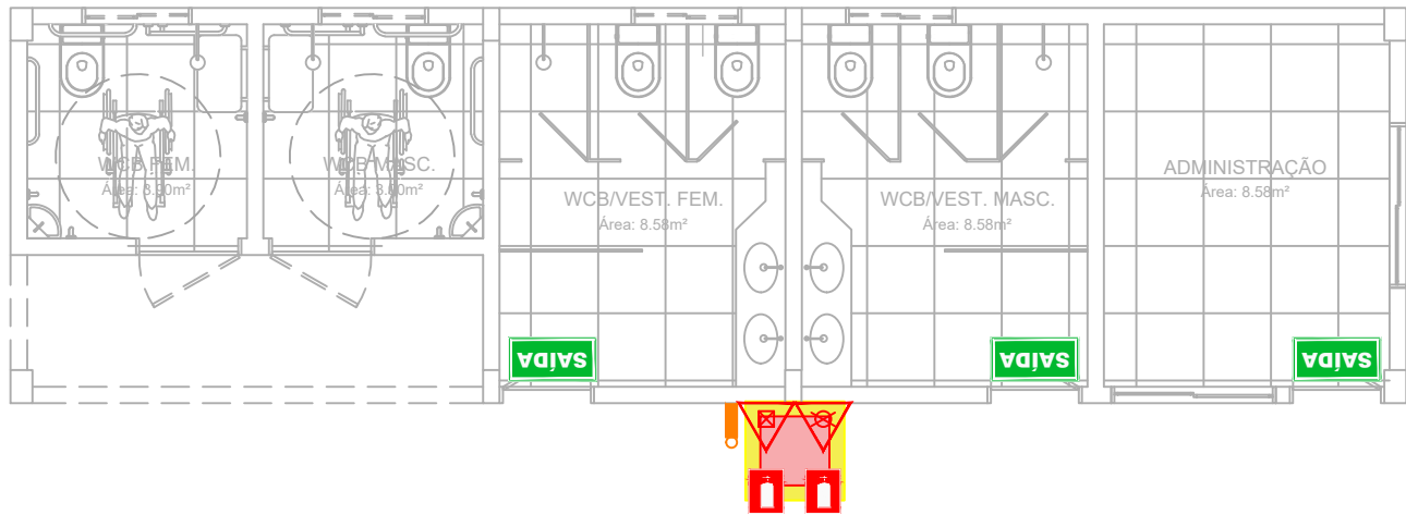
Planta Baixa – Administração/Vestiários/WCB PNE escala 1/75
