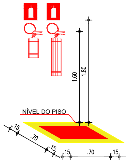
DETALHE EXTINTOR - INSTALAÇÃO PERSPECTIVA
