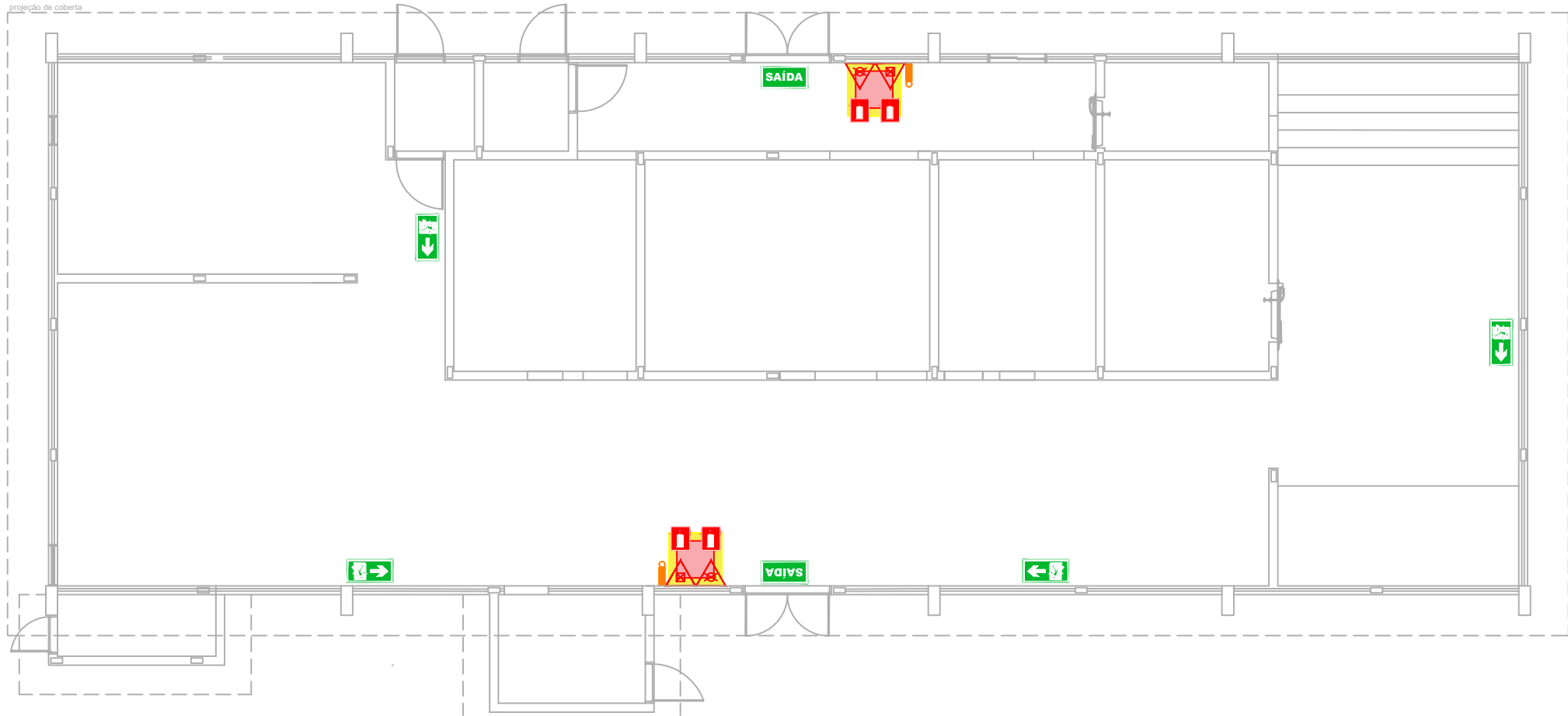
Planta Baixa – Galpão escala 1/100
