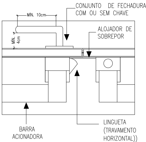
Detalhe 01 escala 1/5
