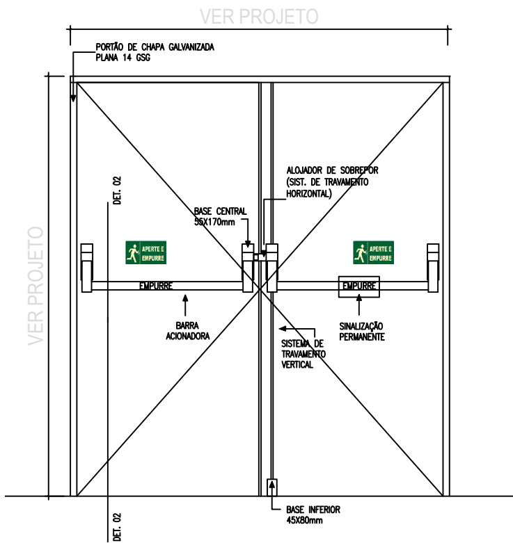
Detalhe em Vista – Portões de Saída de Emergência escala 1/25
