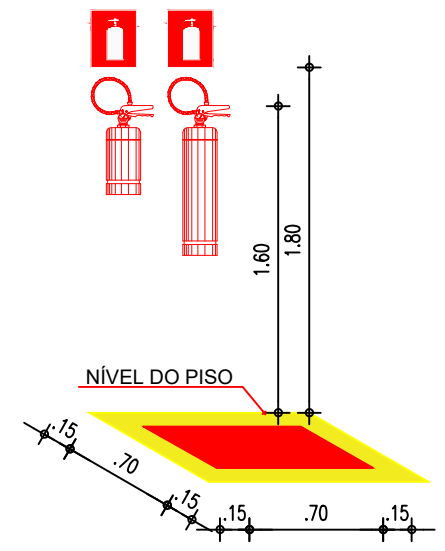
DETALHE EXTINTOR - INSTALAÇÃO PERSPECTIVA
